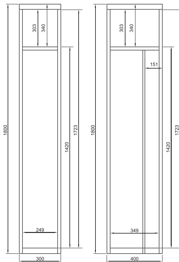
Cotation sans portes, étagères et séparations
