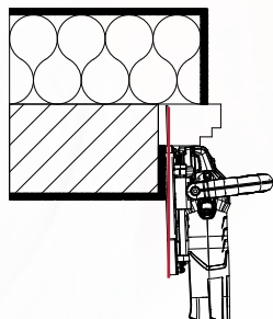
Découpe droite pour des cadres de 70 mm d'épaisseur
