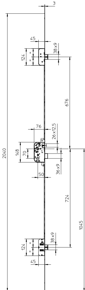
Serrure 3 pts Pènes rectangulaires Longueur 2040 mm
