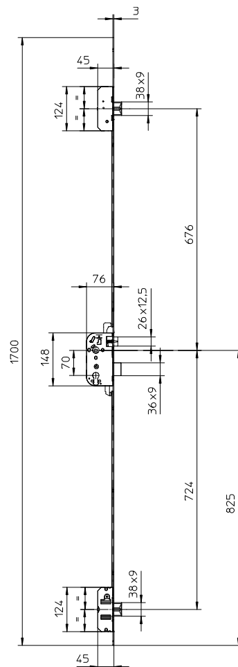
Serrure 3 pts Pènes rectangulaires Longueur 1700 mm
