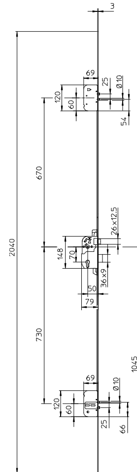
Serrure 3 pts 4 pènes cylindriques Longueur 2040 et 1700mm
