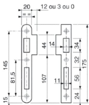
1915 : Gâche plate ép.: 1,5 mm - 2 mm
