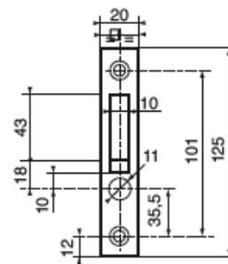
1960 : Gâche plate ép.: 2 mm
