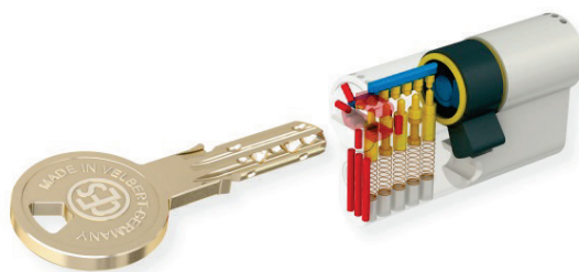
Cylindre WSM5 A2P1* brevet 2030, 4 clés
