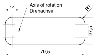
Milling groove Fräsbild
