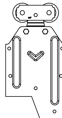
Monture droite Right hanger
