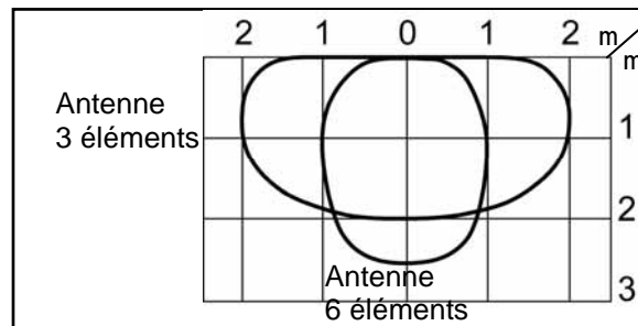
Pour obtenir le lobe étroit, utiliser l'antenne à 6 éléments
