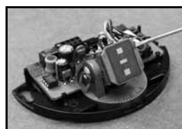
Retirer délicatement l'élément de fixation ainsi que l'antenne lobe large.
