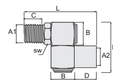
raccord fileté
