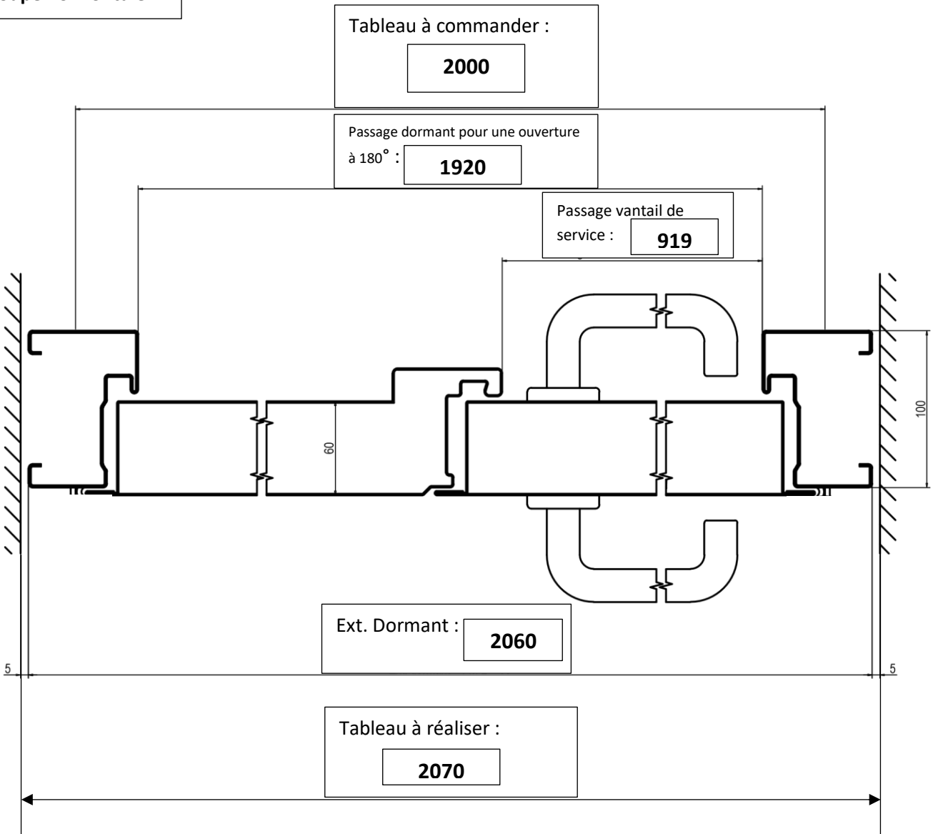
Coupe horizontale
