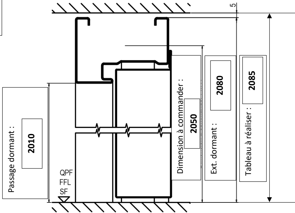
Coupe verticale
