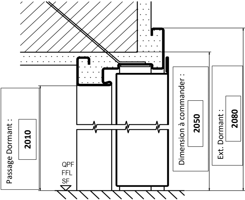
Coupe Verticale
