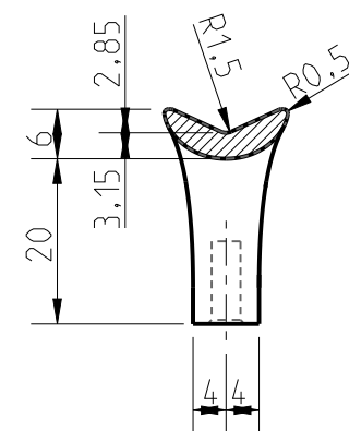
SEZIONE AA-AA
