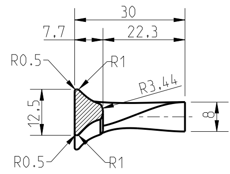
SEZIONE AB-AB
