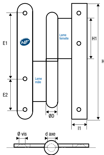
Paumelle gauche
