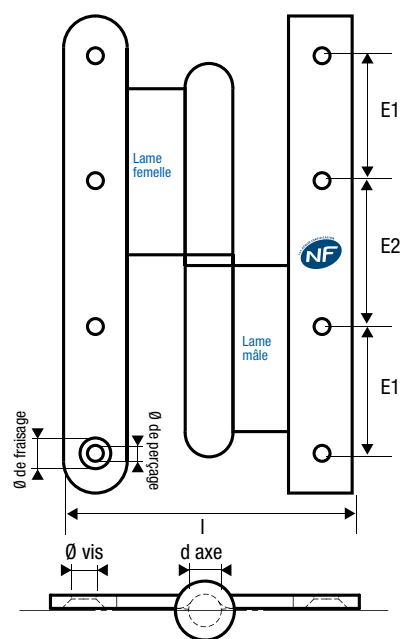
Paumelle droite
