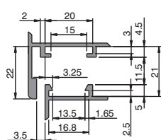
Noeud type 2
