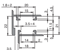
Noeud type 1
