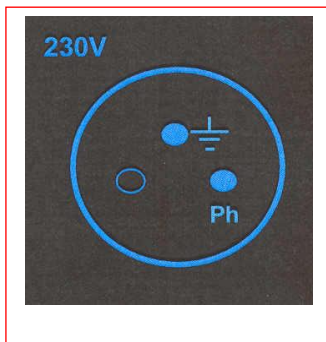
Terre connectée Phase à droite 230 V
