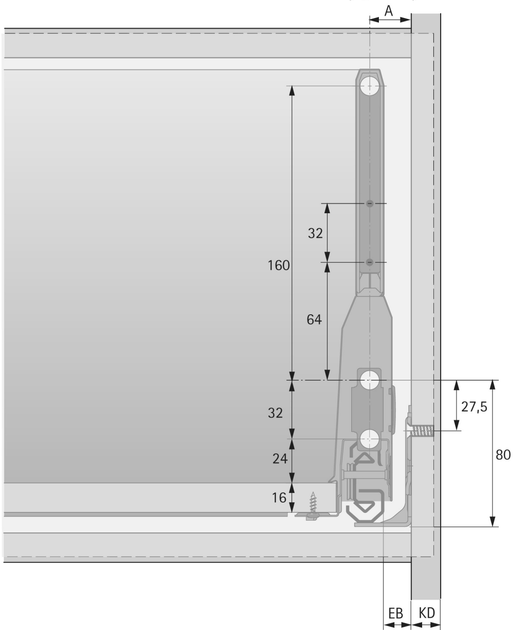
Perçage de façade
