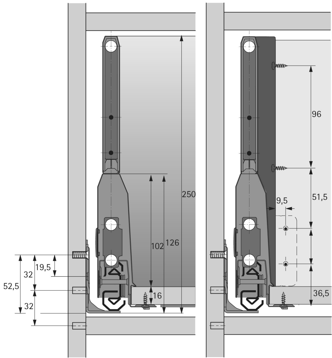
Paroi arrière en acier
