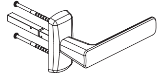
Béquille extérieure sur rosace pour barreur ABLOY Entraxe 92 mm (compatible avec serrures EL/MP électriques)
