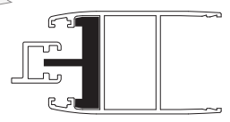
Adaptation avec barrette plate
