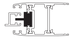
Adaptation avec barrette à tête
