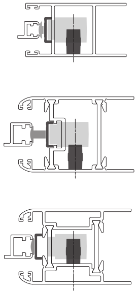
Exemples de réglages du boîtier central
