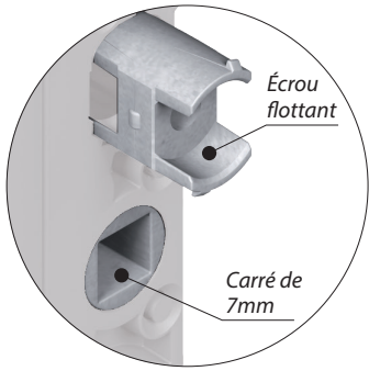
Vis de réglage du crochet
