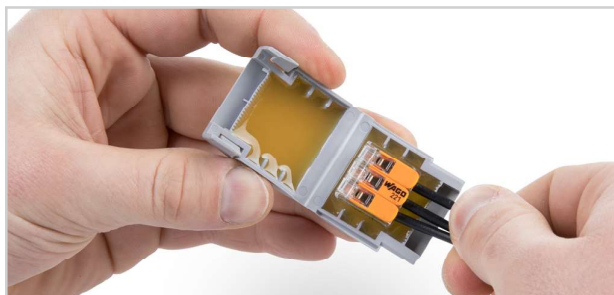
Placez le connecteur câblé dans la Gelbox.
