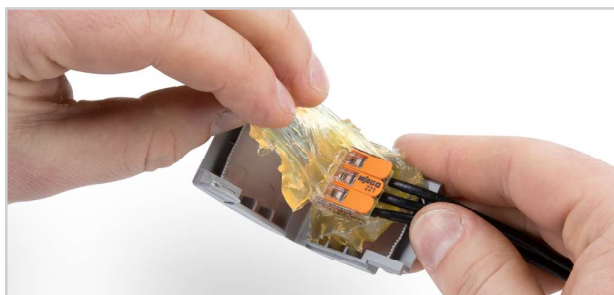
Modifiez simplement les circuits : Ouvrez la Gelbox, retirez le gel du connecteur, ouvrez les leviers du conducteur et connectez les nouveaux composants au câble.
