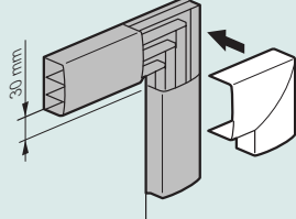
Angle plat
