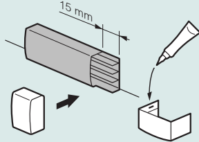
Embout
