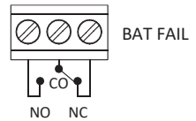
Relais représenté en mode déconnexion batterie(s) seuil bas imminent
